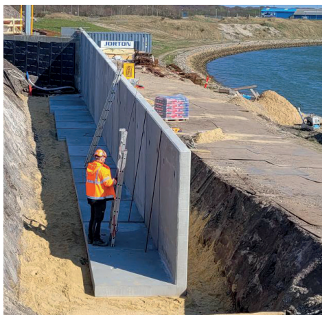
L-elementer og støttemure til Aqtv i Esbjerg Strand.
