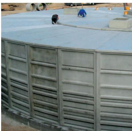
Bassin til afledning af spildevand ved voldsom regn for Forsyning Ballerup A/S.
