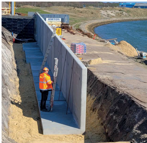
L-elementer og støttemure til Aqtv i Esbjerg Strand.
