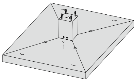
Fundament til tagkonstruktion ved lade-standere.
