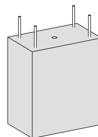
Fundament til ladestander med opragende gevindstænger.
