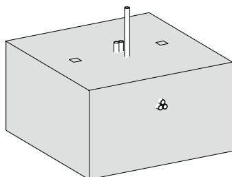
Fundament til fx master med afgang- og ankomstskærme med kabelrør til el.
