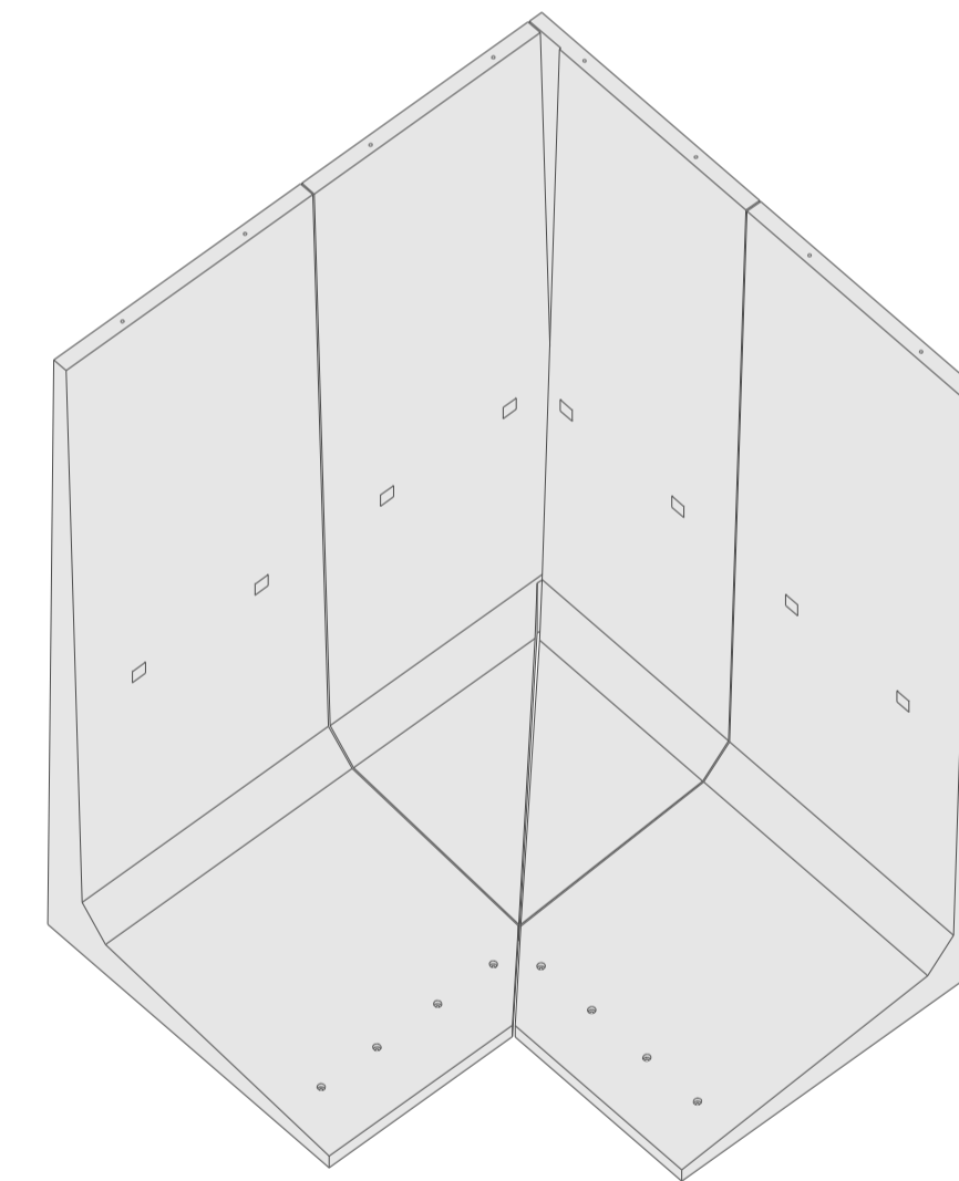
550L Plan Hjørnesamling
