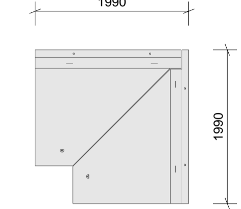
360L Plan Hjørnesamling
