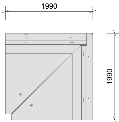
400L Plan Hjørnesamling
