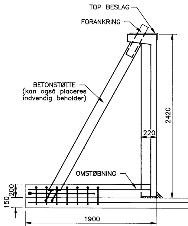
SNIT A-A
