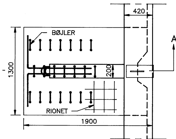
PLAN omstøbning ved støtter
