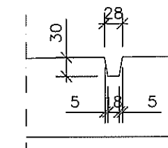
Detalje C
