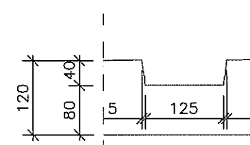
Detalje A
